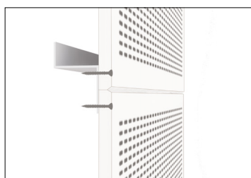
KANT B (Avfasettkant). Synliga skarvar. Passar till Globe.
